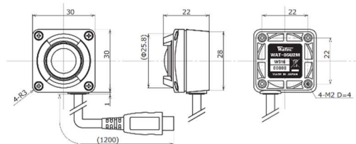
主要寸法図
